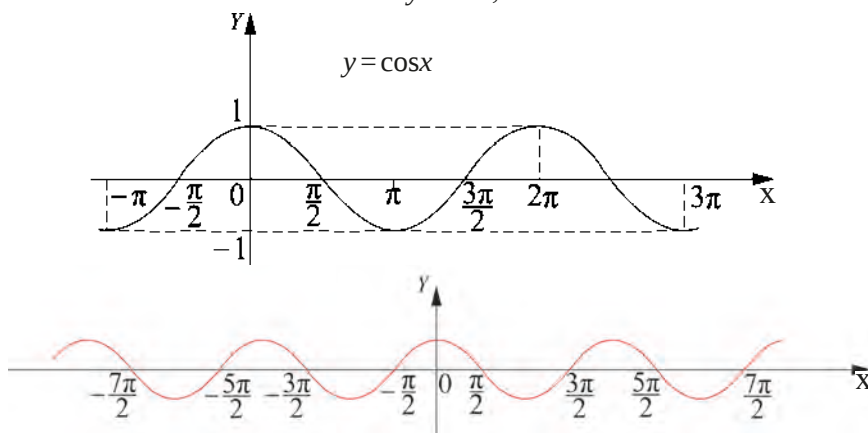
Рис.15. y = \cos x , x \in \mathbb{R} .
