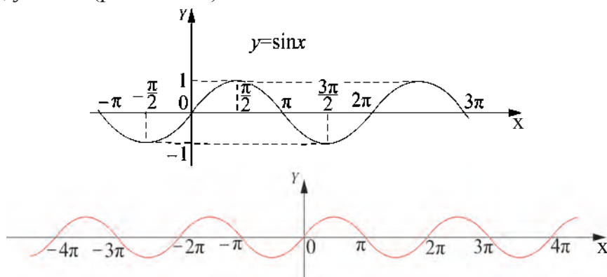
Рис.14. y = \sin x , x \in \mathbb{R} .
