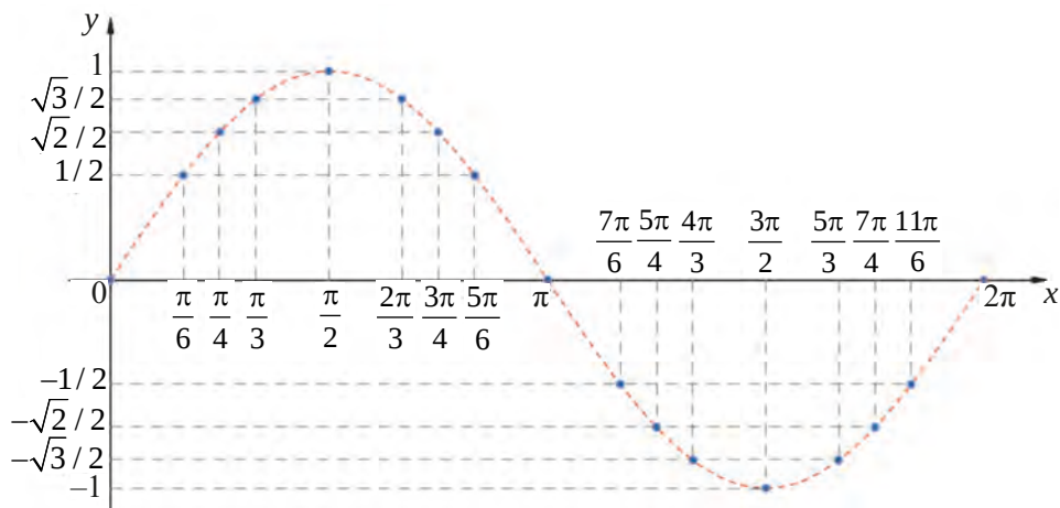
Рис. 12. y = \sin x , 0 \leq x \leq 2\pi .
